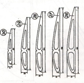
ŽEBRA VÍŠKOVKY - VŠECHNY VÝŘEZY 2x2
