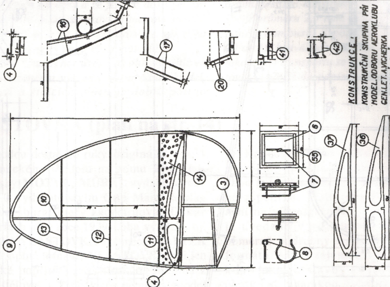
ŽEBRA NOSNÉ PLOCHY VÝŘEZY 2x2, 2x3
